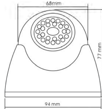
External dimensions unit:mm
